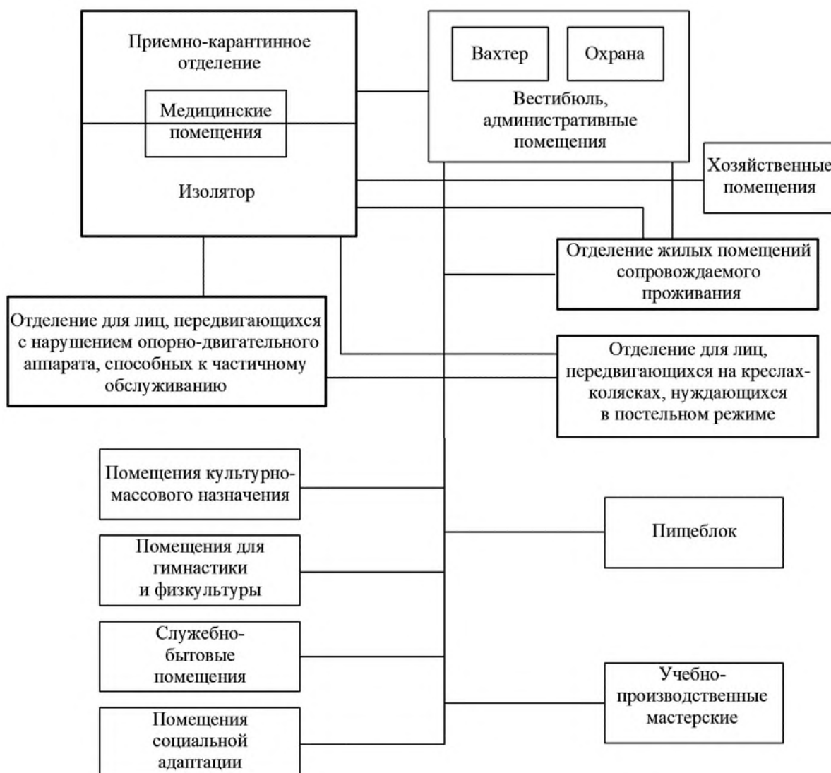
Рисунок А.1 – Схема взаимосвязей жилых групп и помещений дома-интерната со специальным отделением и отделением жилых помещений сопровождаемого проживания
